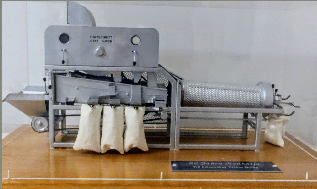
Petkus-lajittelijan pienoismalli lasivitriinissä 60 vuotta täyttävälle Hankkijalle koneiden valmistajalta v. 1965
